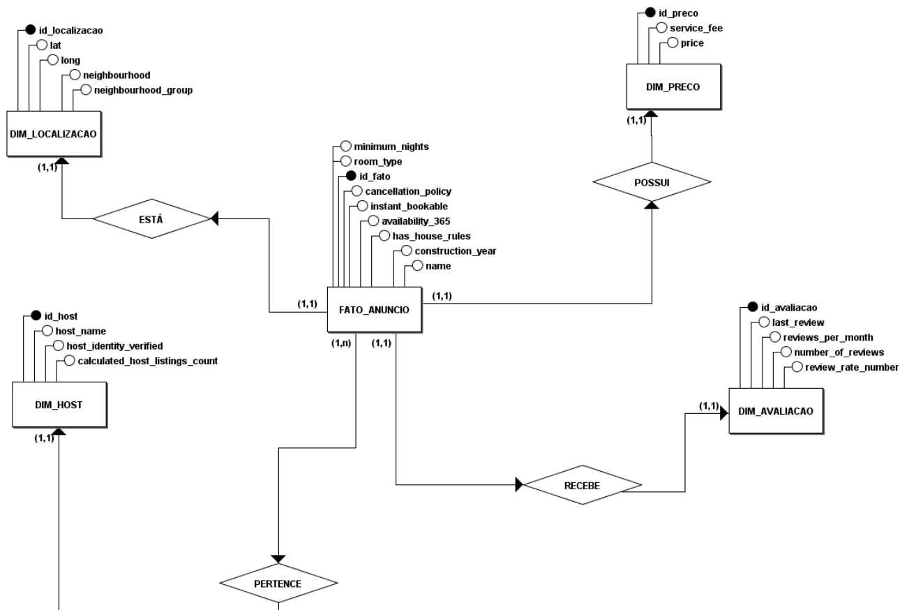
Diagrama Lógico de Dados (DLD)
